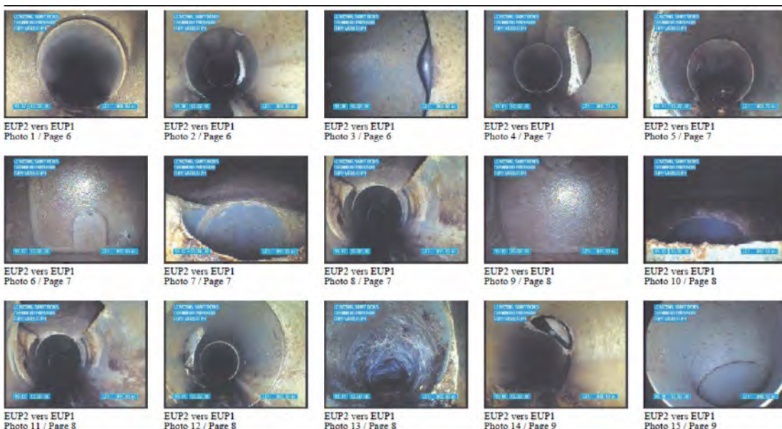
Inspection vidéo d'une canalisation.
